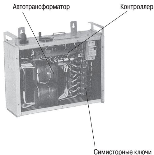
Рис. 8. Устройство стабилизатора
